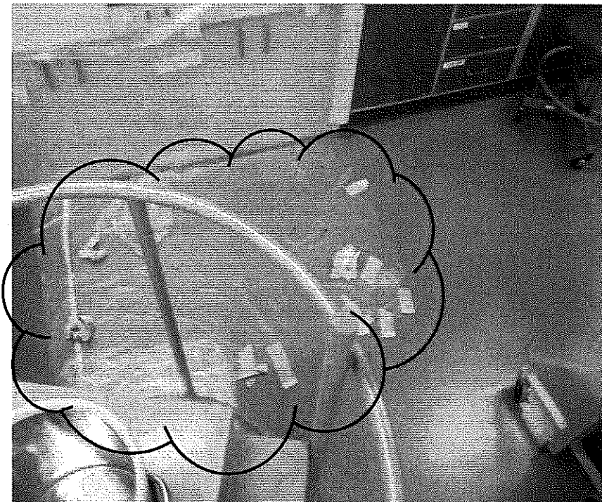
図4 核燃料物質と思われる粒子の主要な飛散場所
