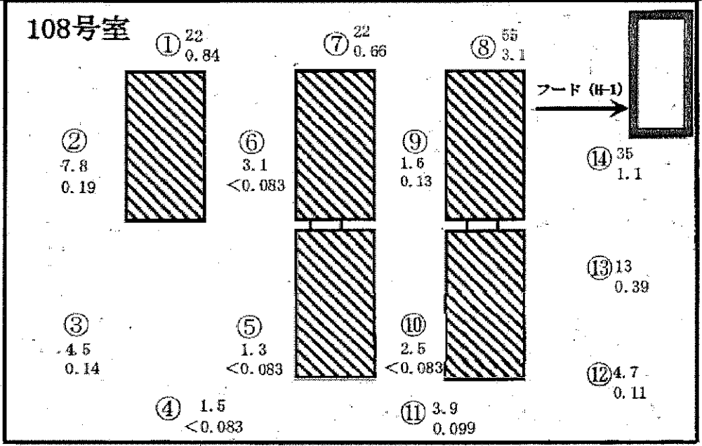
図2 表面密度測定結果
